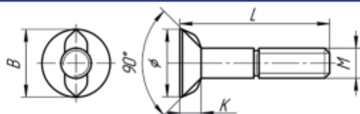
БОЛТ КОНУСНЫЙ С 2-мя ПЛОСКИМИ ГРАНЯМИ
