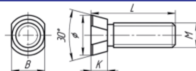
БОЛТ КОНУСНЫЙ С 1-ой ПЛОСКОЙ ГРАНЬЮ
