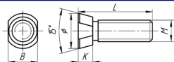
БОЛТ С 2-мя УСАМИ ISO 5713
